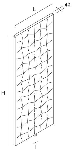
Modèle standard
