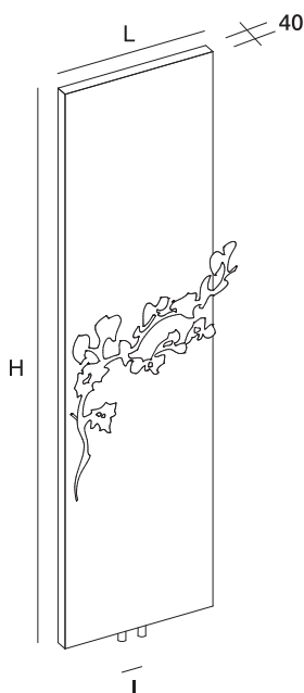
Modèle standard
