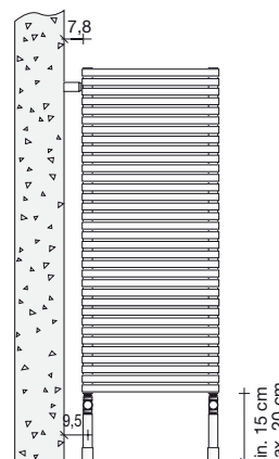
Supports à bras MURAL
