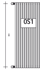
Entraxe l=H-3,4 cm
