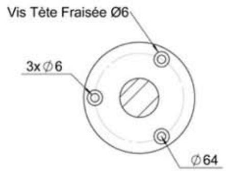
COUPE B-B ECHELLE 1 : 2
